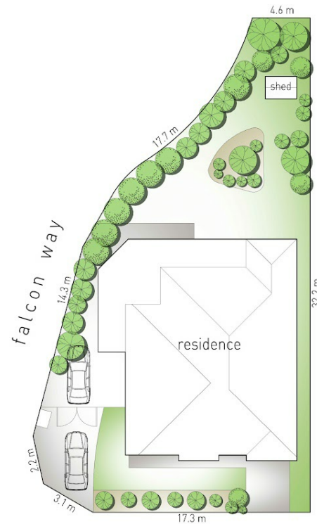
falcon way site plan
